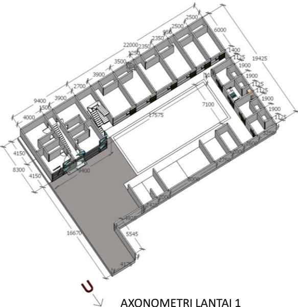
AXONOMETRI LANTAI 1
