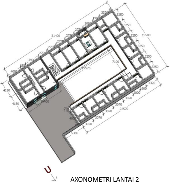
AXONOMETRI LANTAI 2
