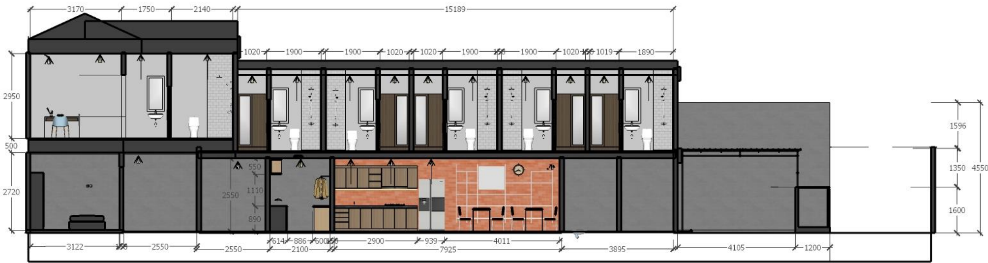
GAMBAR TAMPAK POTONGAN P5
