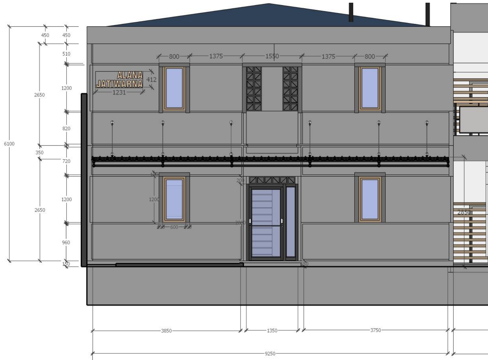
TAMPAK FASAD BANGUNAN A
