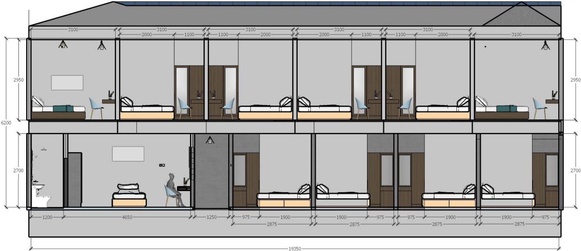
GAMBAR TAMPAK POTONGAN P4
